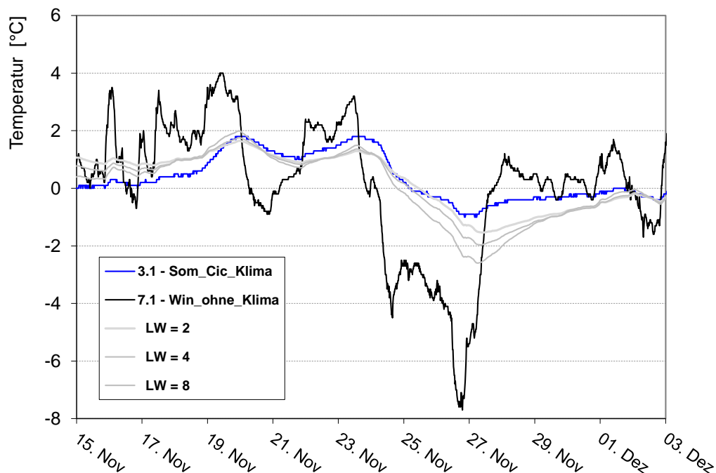
Abb. 131 Vergleichende Darstellung der Temperaturmodellierungen mit Luftwechszelzahlen LW = 2, LW = 4 und LW = 8 mit den Messwerten im ciccum® Winterschutz. Die schwarze Kurve entspricht Umgebungsluft.
