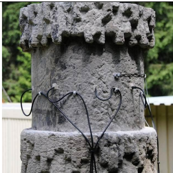
Abb. 116 Digitaler Fühler für Luftfeuchte und Temperatur
