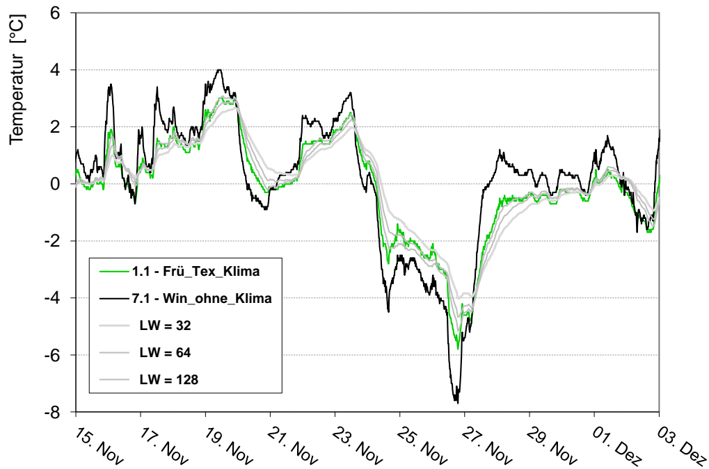
Abb. 130 Vergleichende Darstellung der Temperaturmodellierungen mit Luftwechszelzahlen LW = 32, LW = 64 und LW = 128 mit den Messwerten im Textilien Winterschutz. Die schwarze Kurve entspricht Umgebungsluft.
