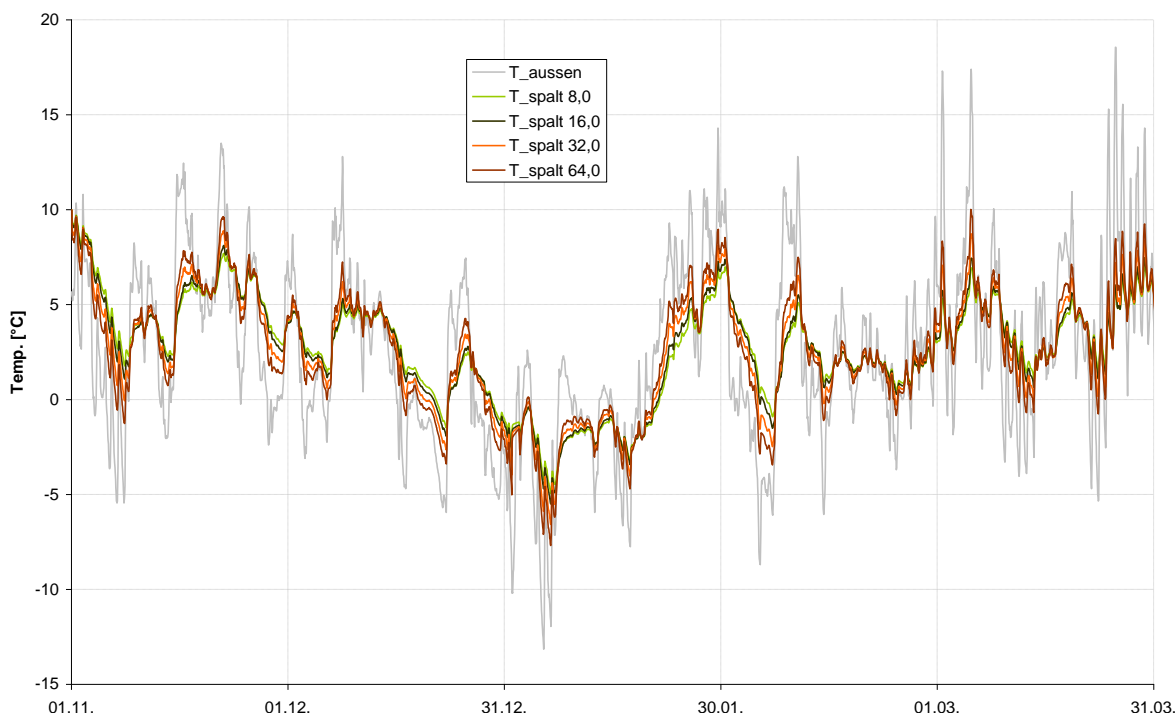
Abb. 126 Temperaturverlauf bei unterschiedlichen Luftwechselzahlen unter der Einhausung
