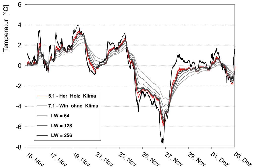
Abb. 132 Vergleichende Darstellung der Temperaturmodellierungen mit Luftwechselzahlen LW = 64, LW = 128 und LW = 256 mit den Messwerten unter der Holztafeleinhausung. Die schwarze Kurve entspricht Umgebungsluft.
